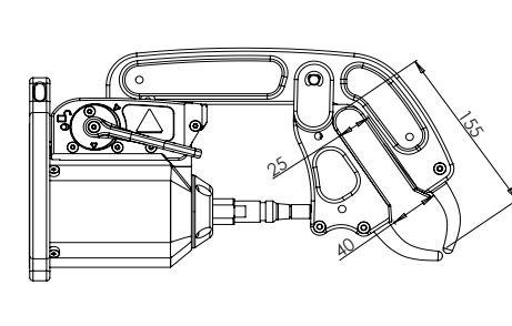
G7 - 022829 4 bar / 150 daN
