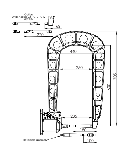
G6 - 022812 8 bar / 550 daN
