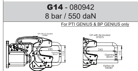
G9_X1 - 022881 8 bar / 550 daN
