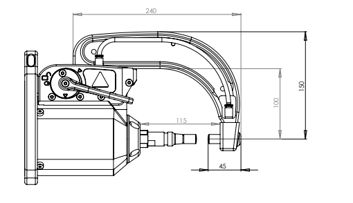
G6 - 022812 8 bar / 550 daN
