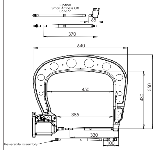
G8 - 022836 8 bar / 550 daN
