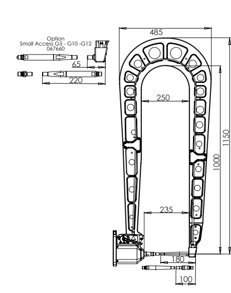
G7 - 022829 4 bar / 150 daN
